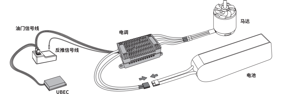
OPTO电调连接图(130A/160A G2)
